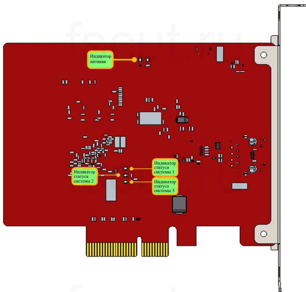
Рисунок 14 Индикаторы BMC228A
