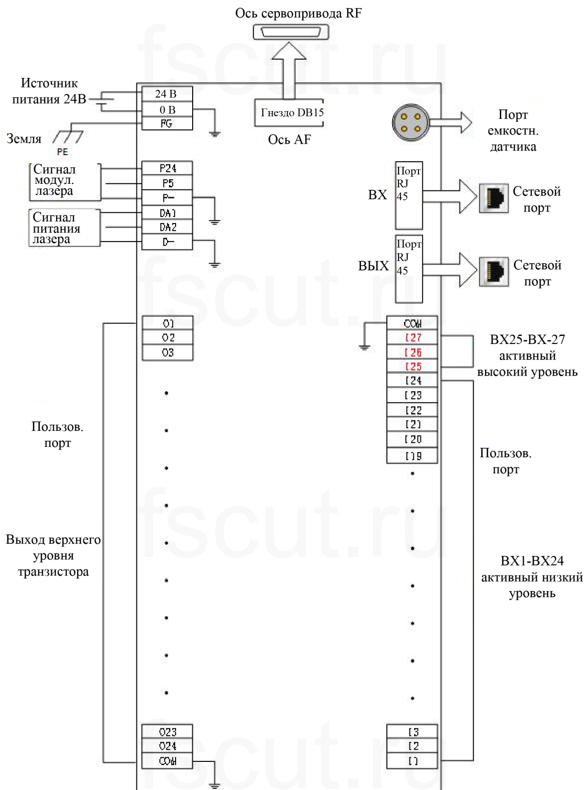
Рисунок 11 Электромонтажная схема BCL4566E
