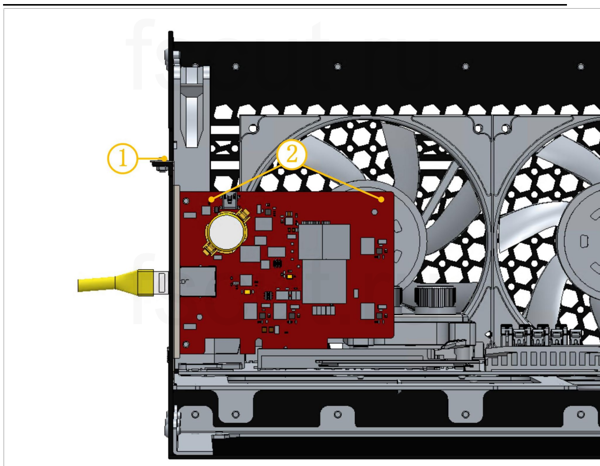
Рисунок 4 Установка платы управления BMC228A Установленная BMC228X представлена ниже.
