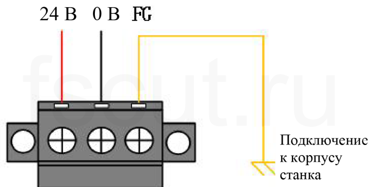
Рисунок 3 Разъем источника электропитания
