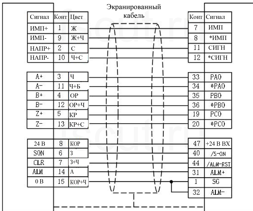
Рисунок 10 Электромонтажная схема сервопривода Yaskawa
