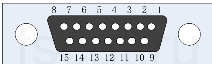
Рисунок 9 Интерфейс сервопривода
