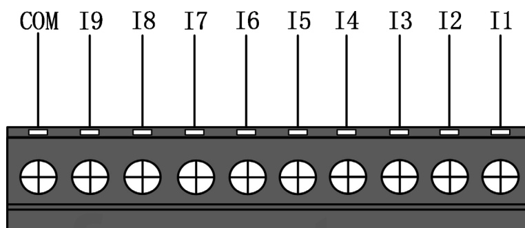
Рисунок 7 Входной разъем
