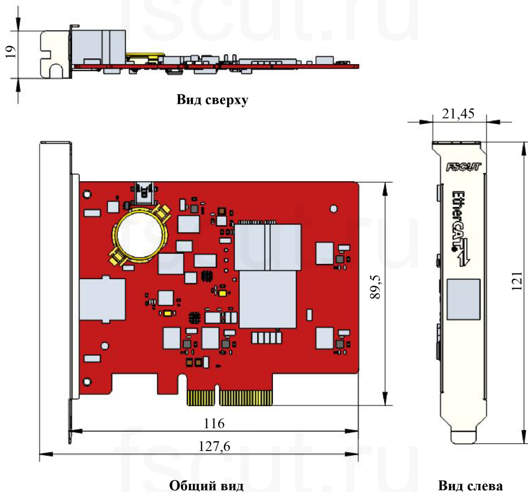
Рисунок 3 Размеры BMC228A
