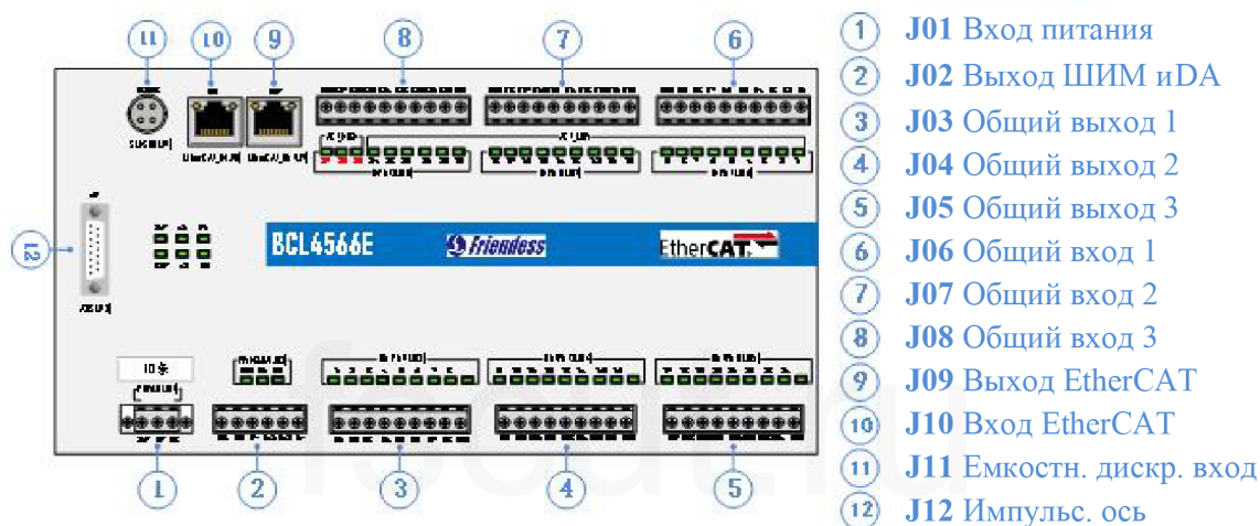
Рисунок 2 Разъемы интерфейса BCL4566E
