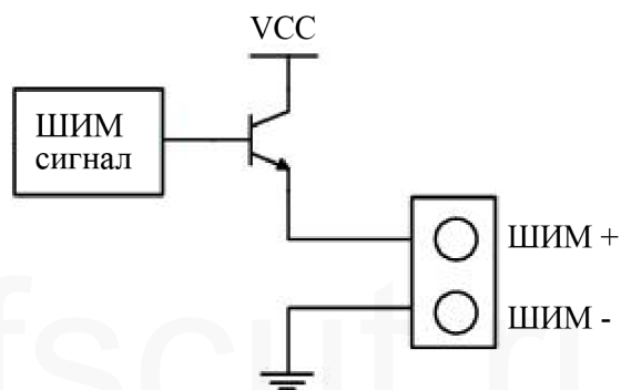
Рисунок 5. Цепь вывода ШИМ
