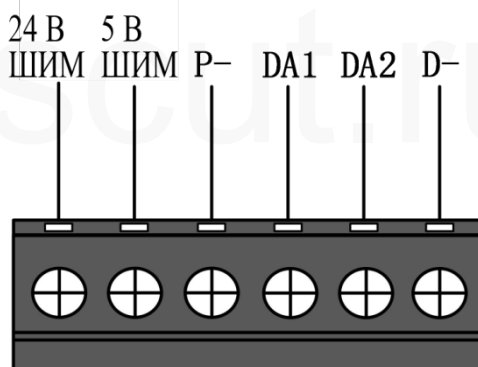
Рисунок 4 Разъемы ШИМ/DA
