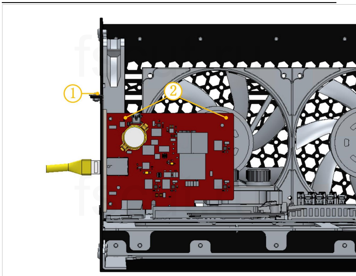
Рисунок 4 Установка платы управления BMC228X
