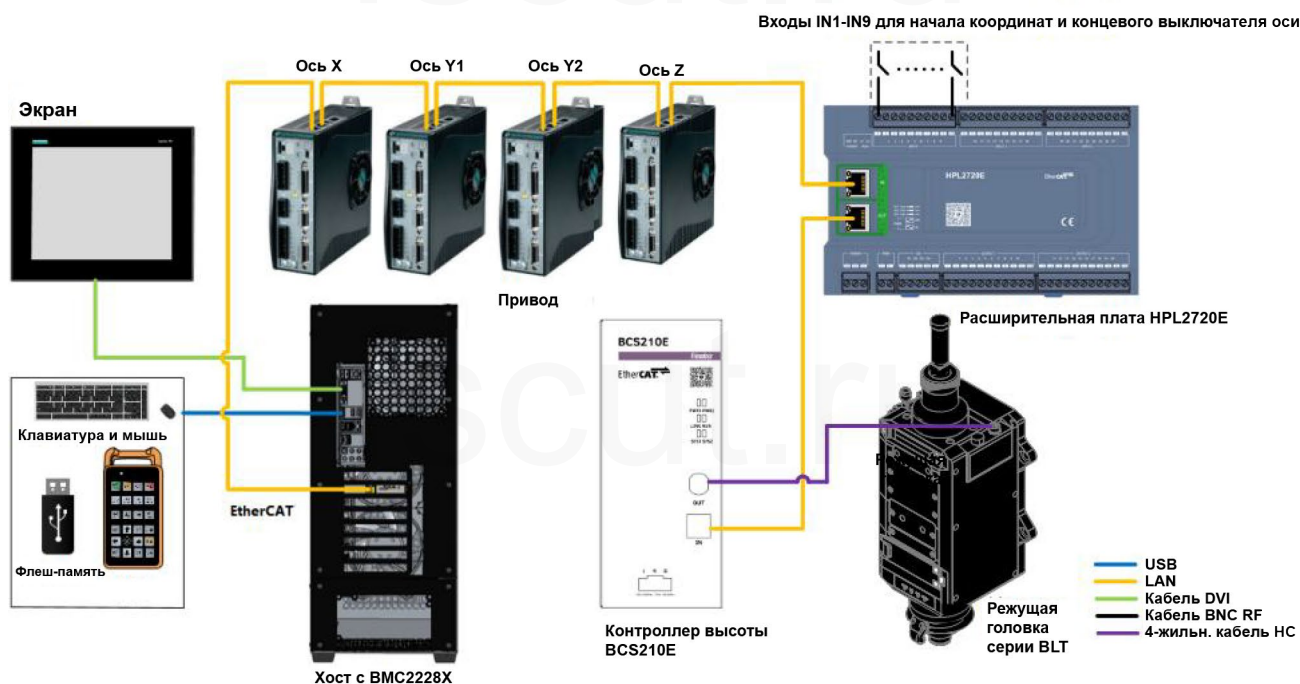
Рисунок 1 Электромонтажная схема FSCUT4000E - Режущая головка серии BLT
