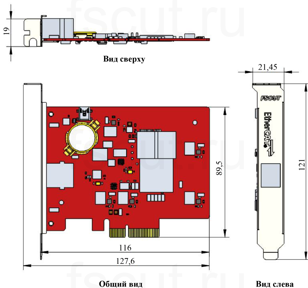
Рисунок 3 Размеры BMC228X
