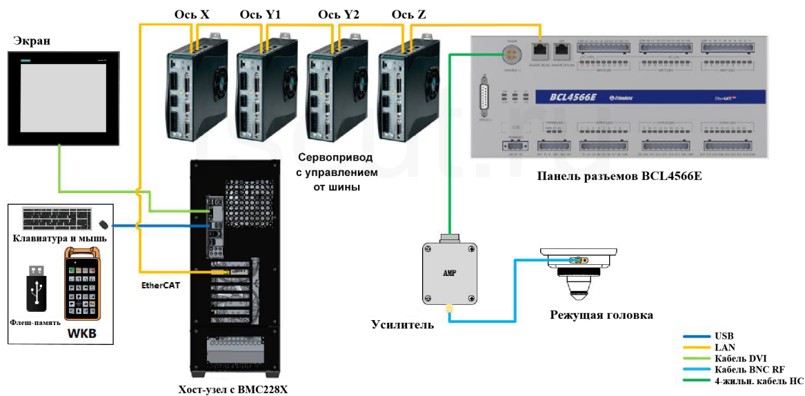
Рисунок 2 Электромонтажная схема FSCUT4000E – другая режущая головка
