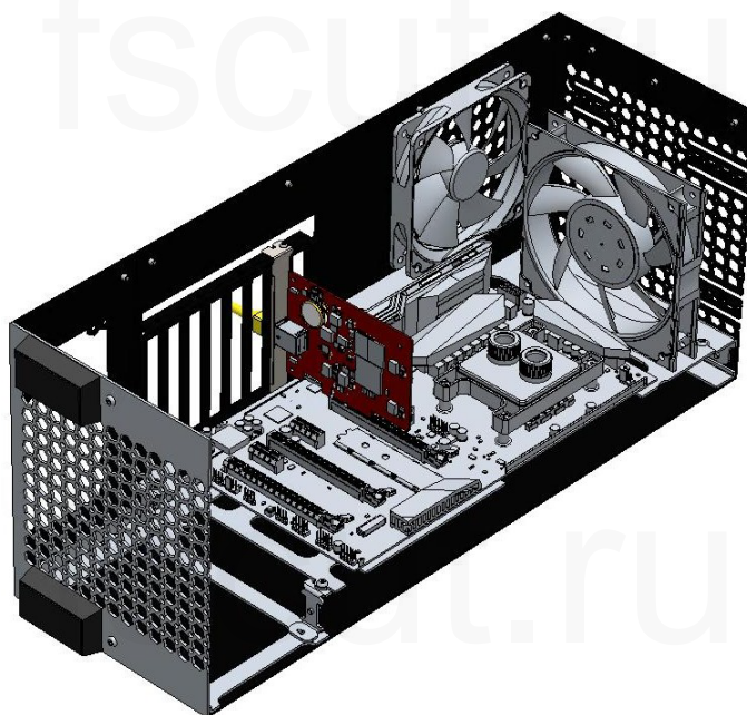
Рисунок 5 Плата управления BMC228X после установки
