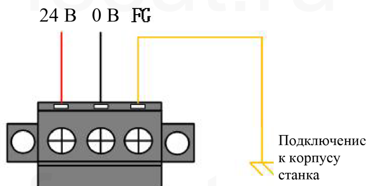
Рисунок 2.3.2 Разъем источника электропитания
