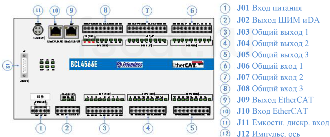
Рисунок 2.3.1 Разъемы интерфейса BCL4566E
